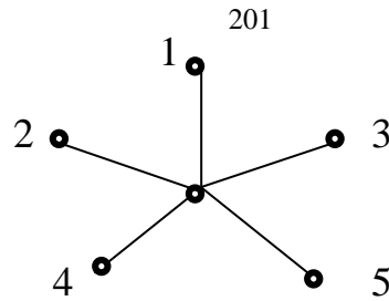
Повний двочастинний граф K_5
