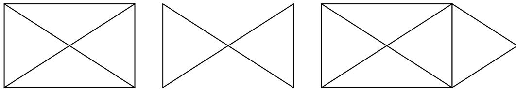
а) неейлерів гра;
