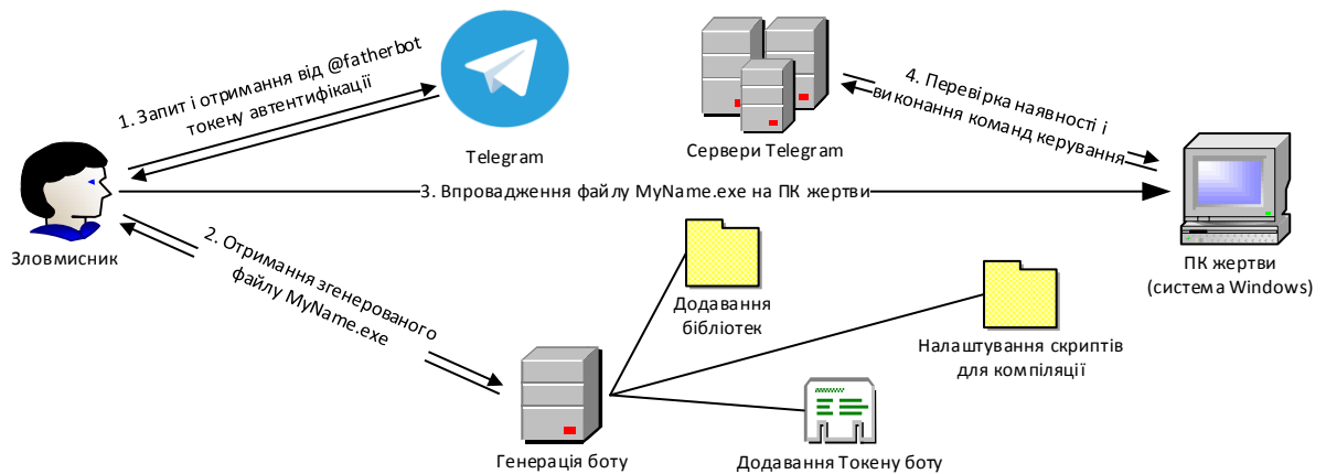
Рис. 1 – Логічна схема прихованого віддаленого доступу до комп'ютерної системи
